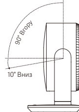
100° Вертикальне коливання
